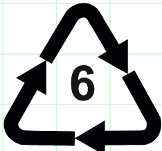
PS Polystyrene
